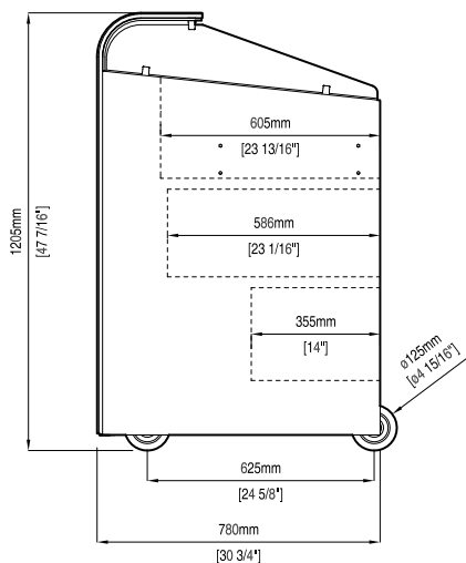
Zij aanzicht
